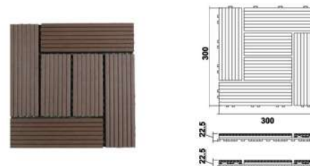
VỈ GỖ NHỰA VIỆT PHÁP 300x300x24 MM KÍCH THƯỚC: 300 x 300 x 24 MM
