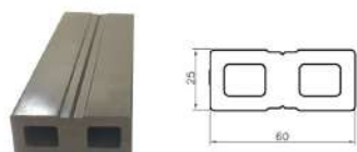
THANH XƯƠNG GỖ NHỰA VIỆT PHÁP BẢN 25x60 MM KÍCH THƯỚC: 25 x 60 MM
