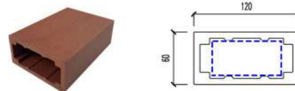
THANH HỘP GỖ NHỰA VIỆT PHÁP BẮN 60x120 MM KÍCH THƯỚC: 60 X 120 MM (*) KÍCH THƯỚC THÉP HỘP: 40 x 80 mm
