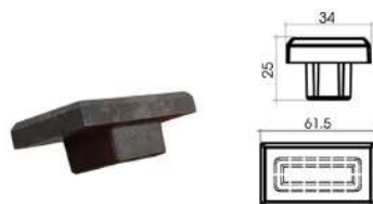
NÚT BỊT GỖ NHỰA VIỆT PHÁP 32x60 MM KÍCH THƯỚC: 32 x 60 MM
