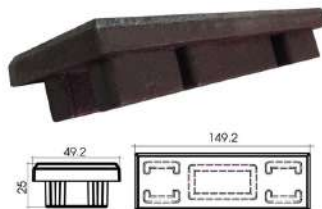
NÚT BỊT GỖ NHỰA VIỆT PHÁP 50x150 MM KÍCH THƯỚC: 50 x 150 MM
