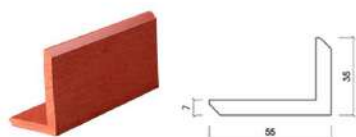
THANH NẸP GỖ NHỰA VIỆT PHÁP BẢN 35x55 MM KÍCH THƯỚC: 35 x 55 MM
